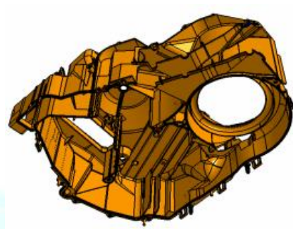
空調大殼體（右）
